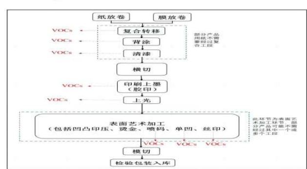
胶印工艺流程图：
