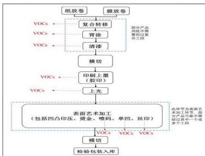
胶印工艺流程图：
