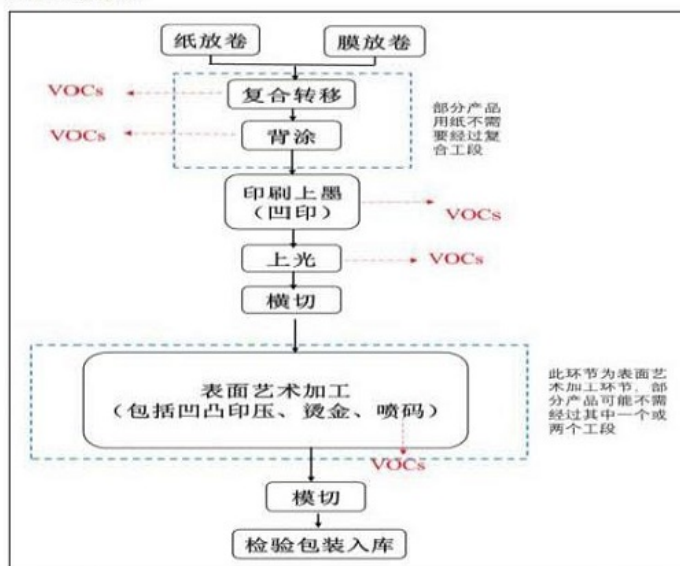
凹印工艺流程图：
